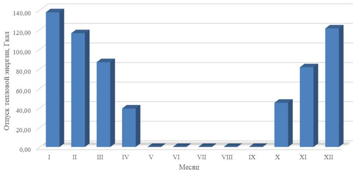
Рисунок 1.3 – Оптимальный температурный график отпуски тепловой энергии по сельской котельной
