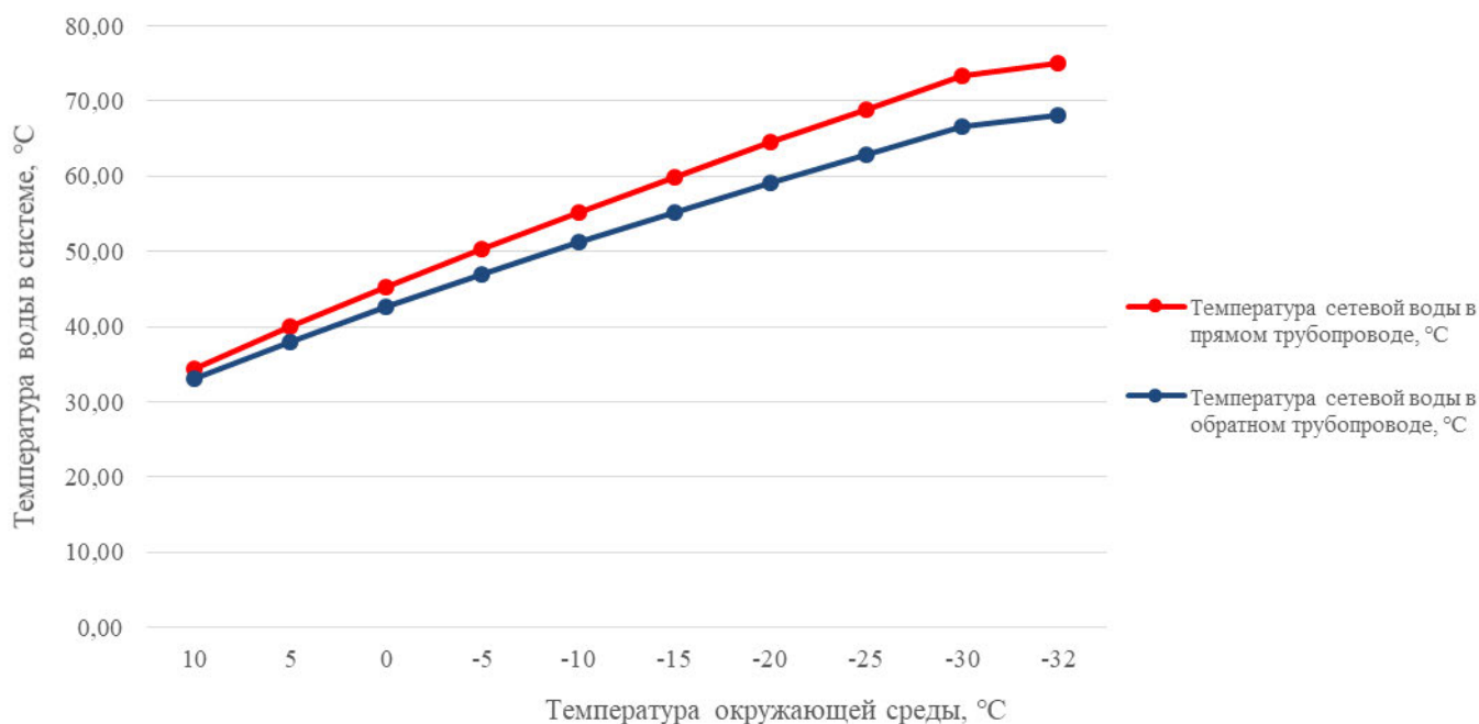
Рисунок 2.2 – График изменения температур теплоносителя котельных (температурный график 75/68°C)
